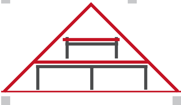
Kehlbalkendach zweistöckig mit zweifach/dreifach stehendem Stuhl
