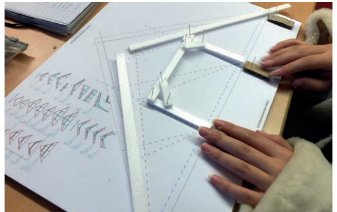
Konstruieren mit Balken aus Polystyrolplatten
